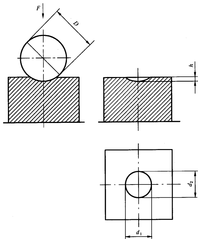
图1 试验原理
